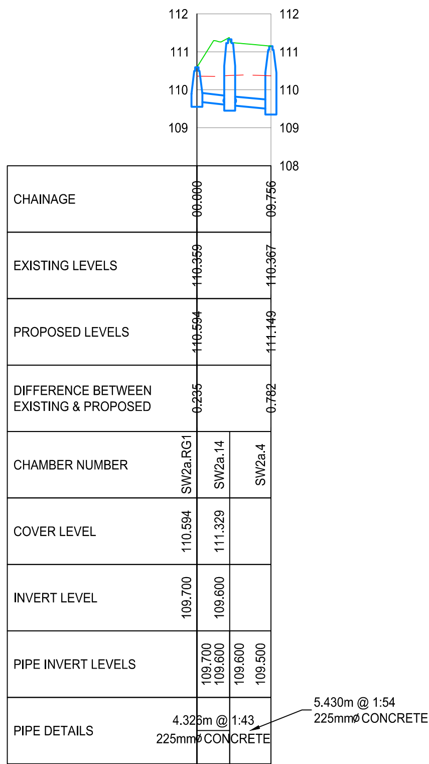
SW LS - 1.16 SCALE: H 1:500,V 1:100. DATUM: 108.000
