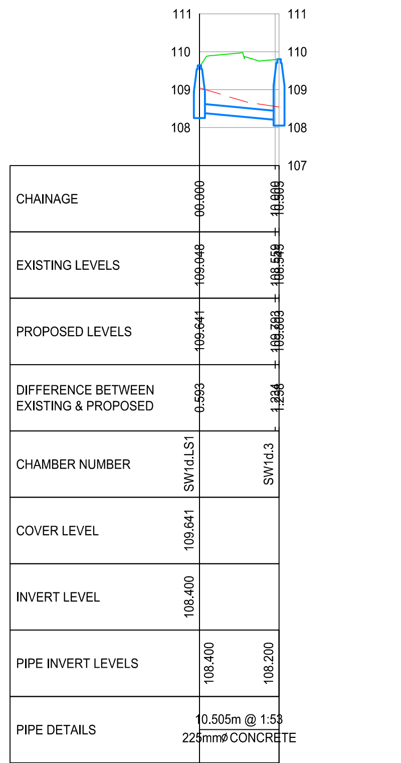
SW LS - 1.17 SCALE: H 1:500,V 1:100. DATUM: 107.000
