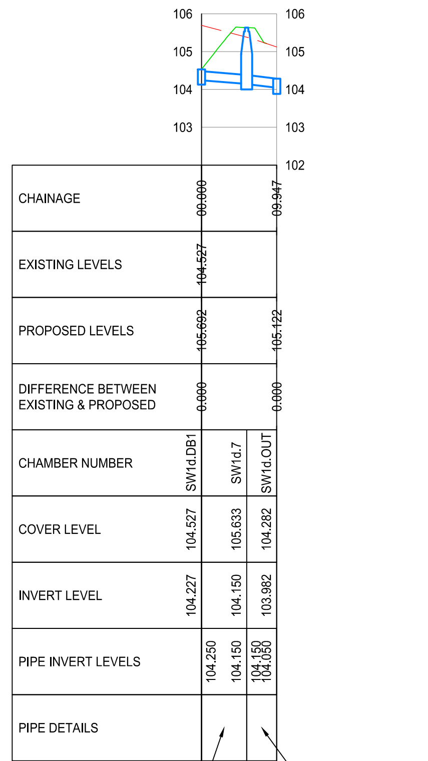
SW LS 1.18 SCALE: H 1:500,V 1:100. DATUM: 102.000
